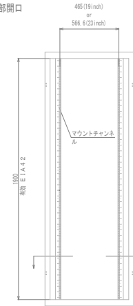
内部開口
