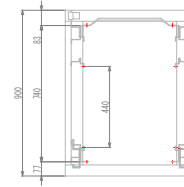
内部開口
